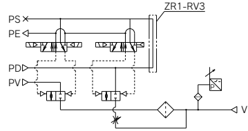
回路例
