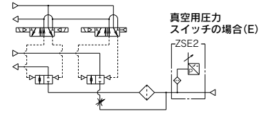
回路図
