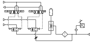
回路図
