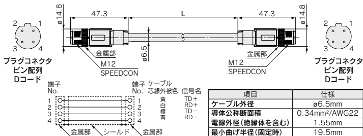
結線図(ストレートケーブル)
