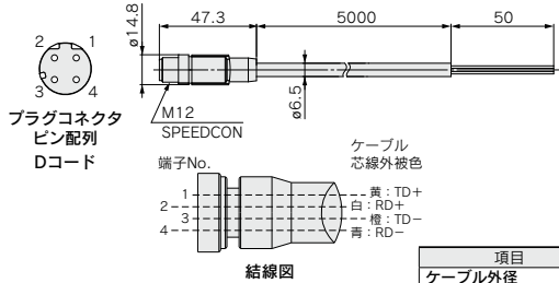
結線図
