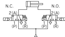
外部パイロット形
