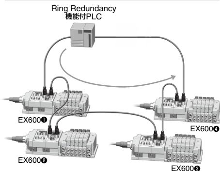
通常時のデータの流れ
