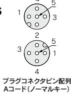
①M12 5ピンプラグ
