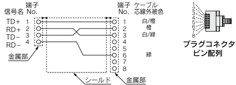
結線図(ストレートケーブル)
