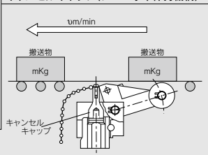
キャンセルキャップ(レバー水平保持機構)
