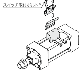
(φ32 D-P3DWA取付例)
