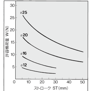
〈図4〉耐横荷重形 / オートスイッチ付
