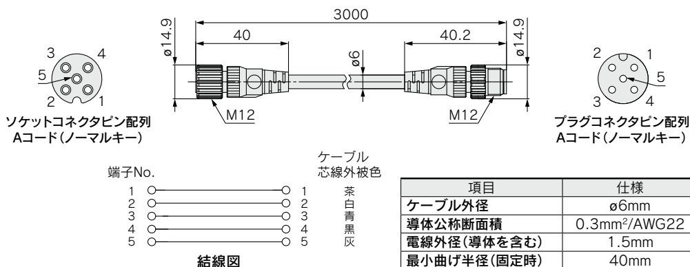
結線図
