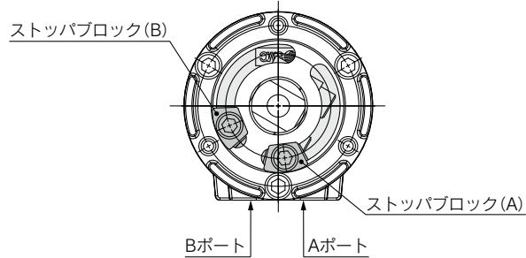
図. 出荷状態(ダブルペーン)
