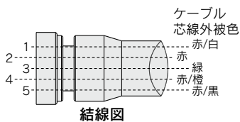
結線図
