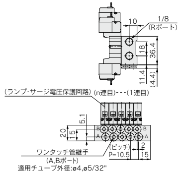
C4, N3□の場合(ワンタッチ管継手内蔵)
