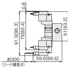
M形プラグコネクタ(M)
