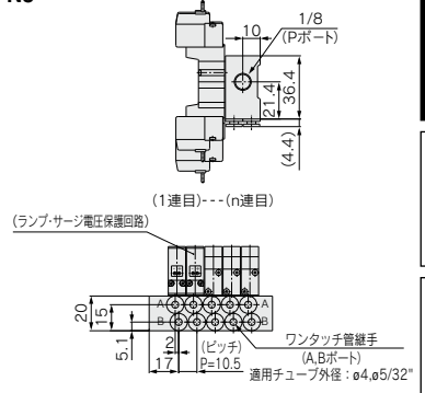
C4, N3□の場合(ワンタッチ管継手内蔵)
