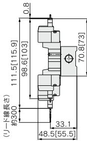
L形プラグコネクタ(L)
