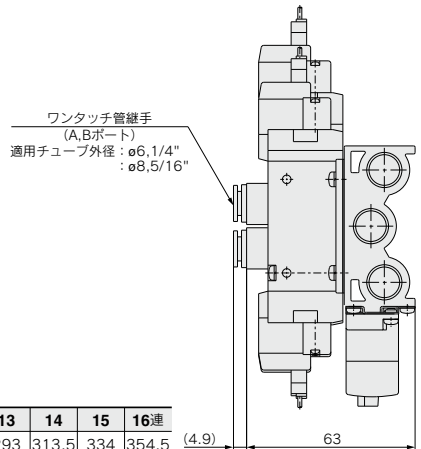
ワンタッチ管継手内蔵形の場合
