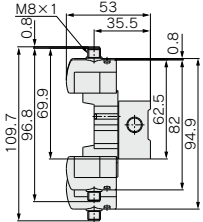
M8コネクタ(WO)
